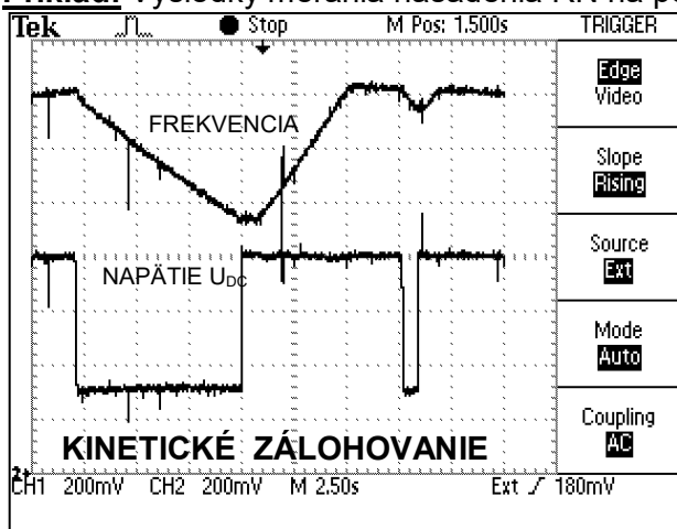
Kinetické zálohovanie meniča pri výpadku napájacieho napätia na motore so zotrvačnikom.
